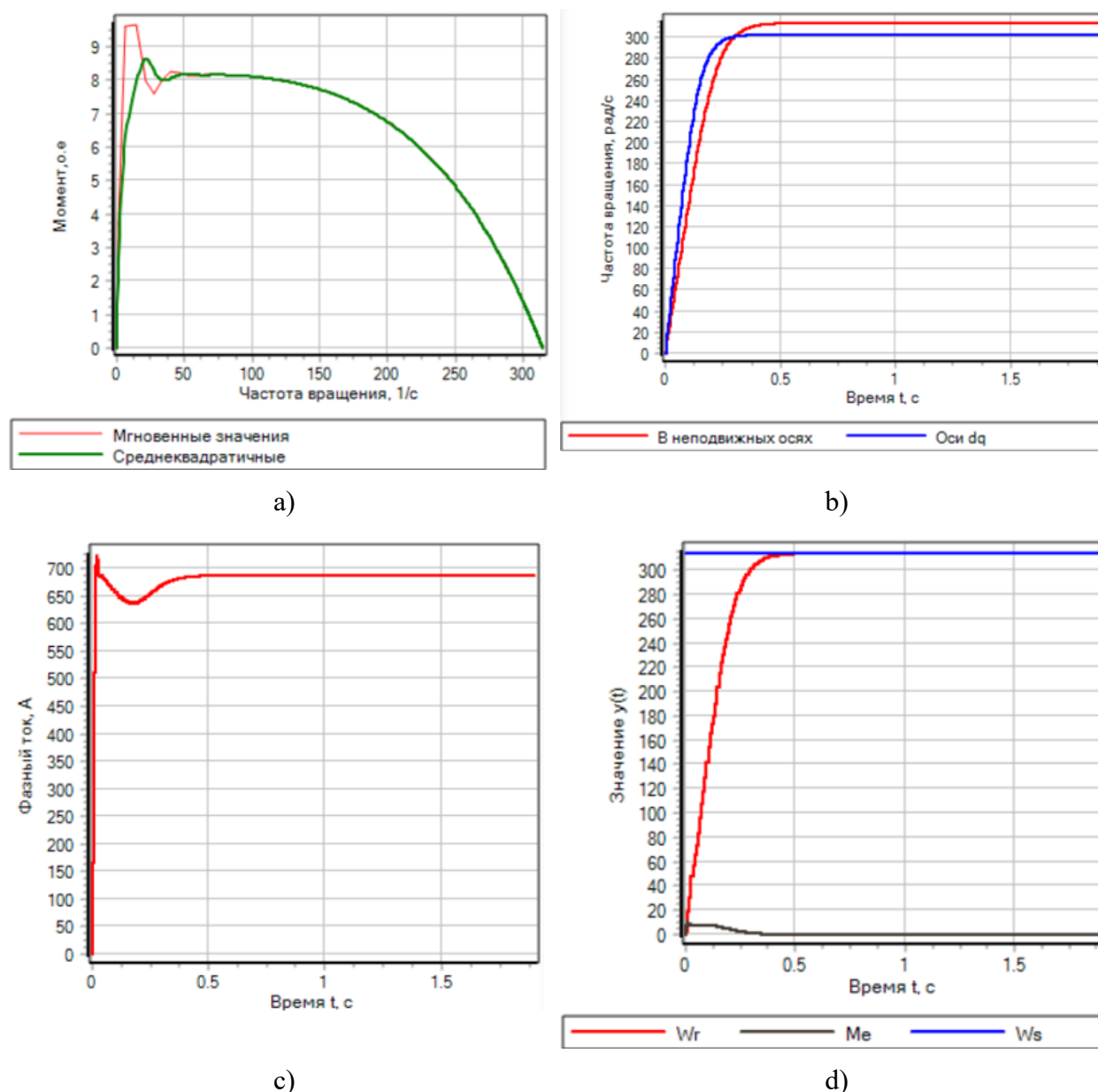
Рис. 5. Имитационное моделирование электродвигателя смесителя комбикорма: а) зависимость момента от частоты вращения, б) частота вращения во времени, в) фазный ток во времени, г) динамика угловой скорости, момента и скольжения
