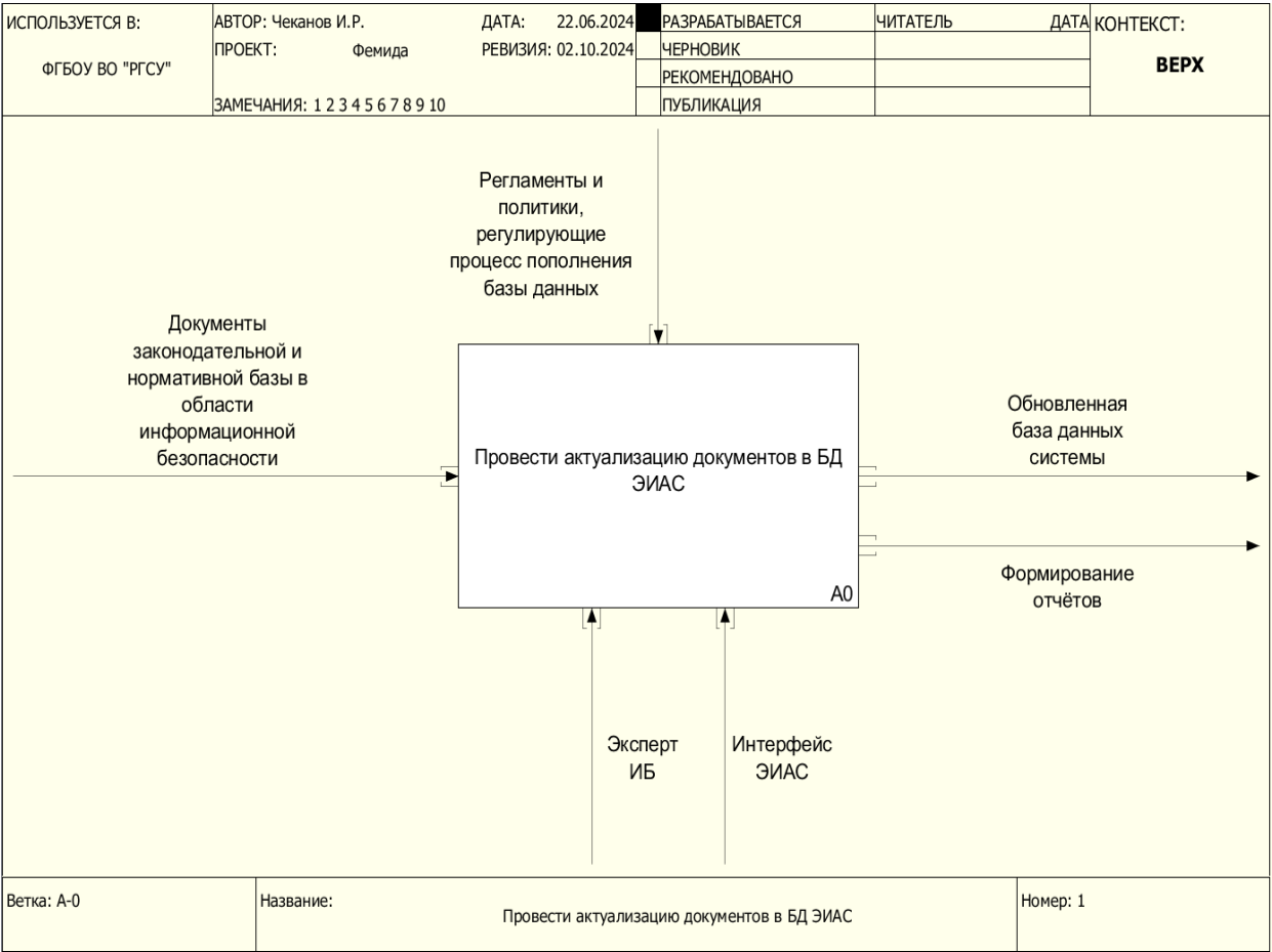
Рис. 1. Обобщенная информационная модель предварительной обработки документов в области ИБ в ЭИАС Fig. 1. Generalized information model of preliminary document processing in the field of information security in the EIAS
